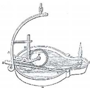
РИС. 4. ► Реконструкция проекта масляного светильника Герона Александрийского
