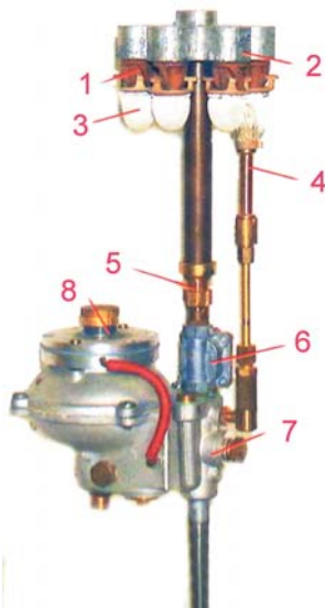
РИС. 11. ► Устройство современного уличного газового ретросветильника
